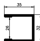
22134 Pystysuora U-profiili
