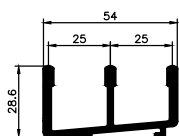
19035 Liukukisko-3
