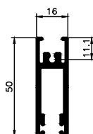
18165 Vaakasuora profiili
