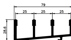
18163 Liukukisko-4
